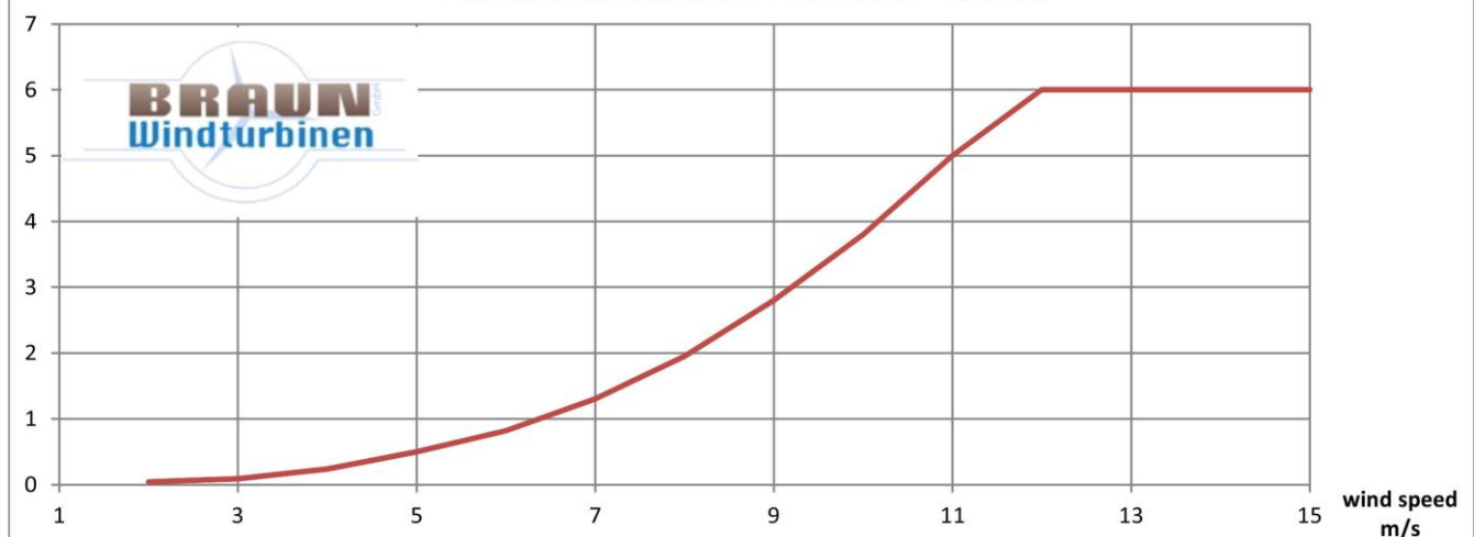
Turbinenkennlinie ANTARIS 4.5kW
